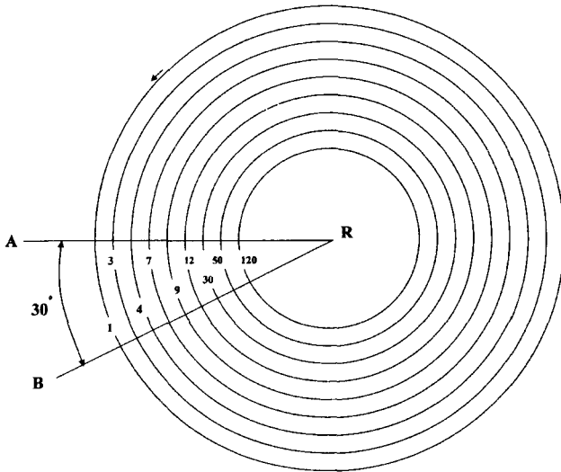
Рис. 1. «Луковичная» система дирекций. Различные дирекции проходят дугу А – В, равную 30°, за различное время
